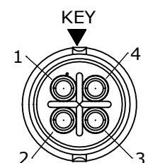
WIRING END W6382-4SG-P-3XX
