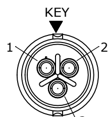
WIRING END W6382-3SG-P-3XX
