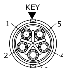
WIRING END W6382-5SG-P-3XX
